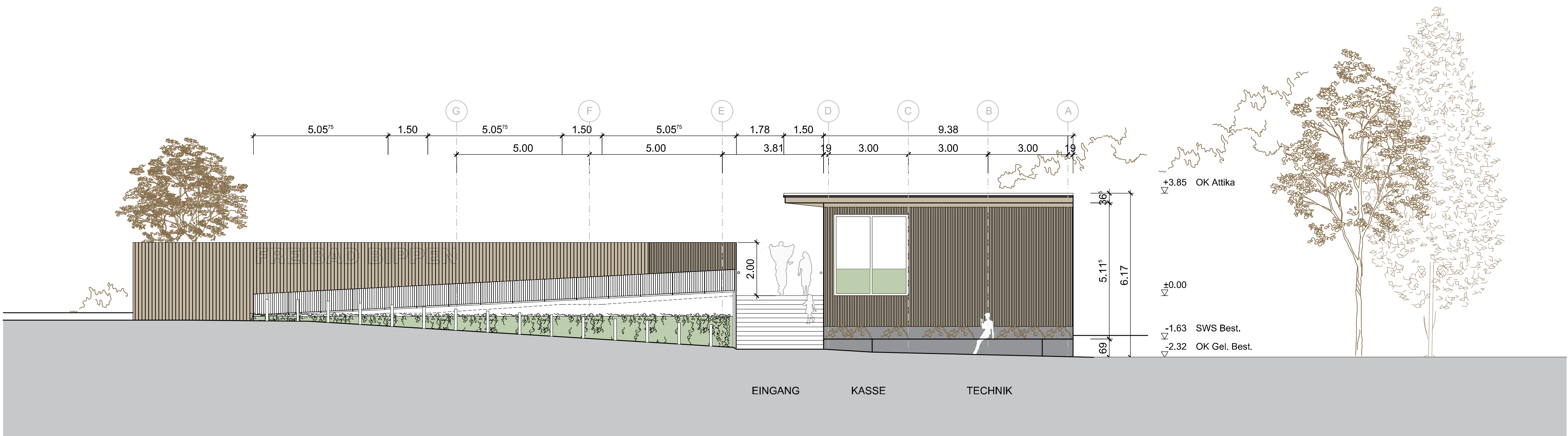
Ansicht Nordost
