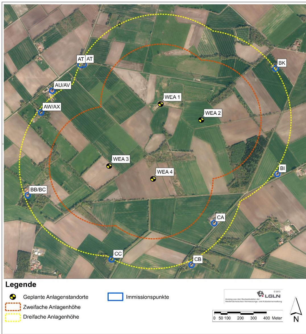
Abb. 7 Lage der untersuchten Wohngebäude zur optisch bedrängenden Wirkung zum geplanten Windpark
