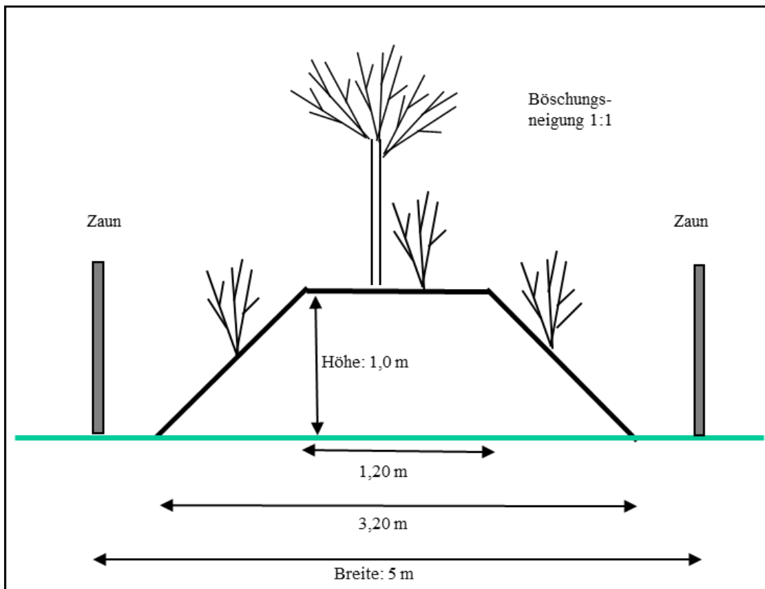
Abb. 31 Wallprofil eines Neuen Kampwalles (Schupp & Dahl, 1992)
