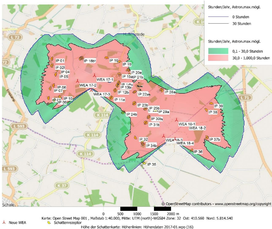
Abb. 6 Schattenwurf Gesamtbelastung unter der Berücksichtigung der Vorbelastung, Kriterium 30 Std. pro Jahr, © Zech Ingenieurgesellschaft
