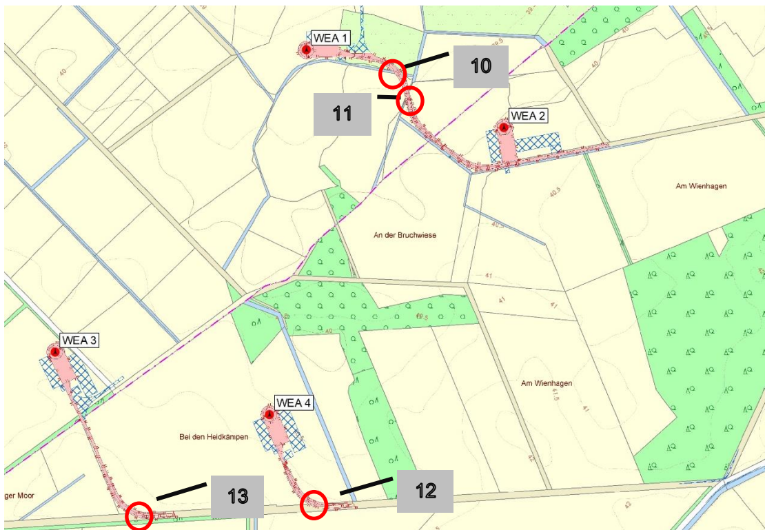
Abb. 19 Lage der notwendigen Grabenquerungen (rote Kreise) (Nummerierung gemäß „Anlage zum wasserrechtlichen Antrag – Übersichtsplan“, Quelle : Agrowea)
